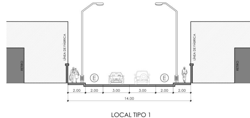
GRAFICO N° 2. Especificaciones Técnicas para el diseño de Vías.
